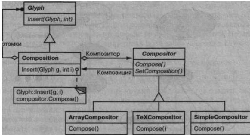
Рис. 2.5. Отношения классов Composition и Compositor
