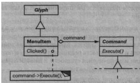
Рис. 2.12. Отношение между классами MenuItem и Command
