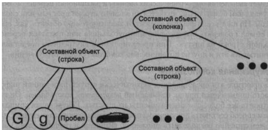
Рис. 2.3. Структура объекта для рекурсивной композиции текста и графики
