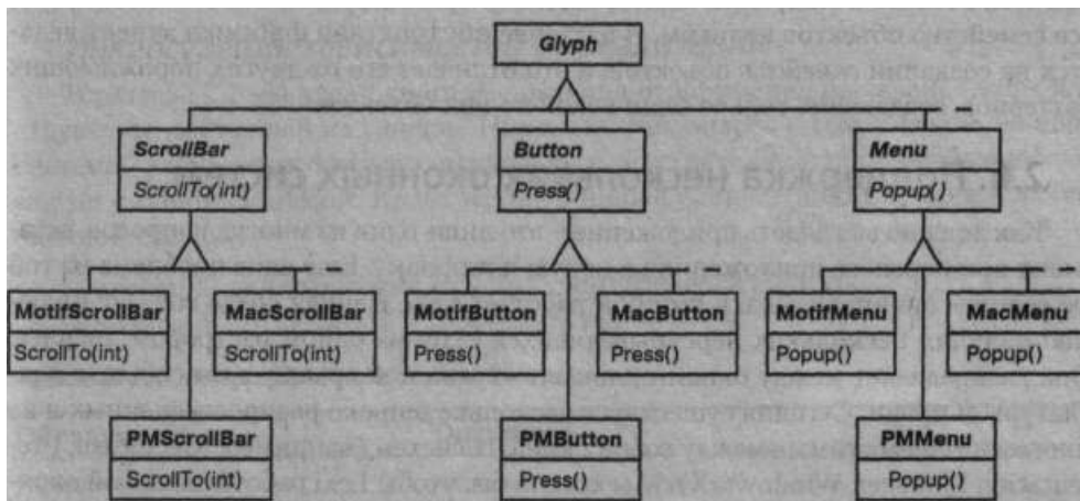
Рис. 2.10. Абстрактные классы-продукты и их конкретные подклассы
