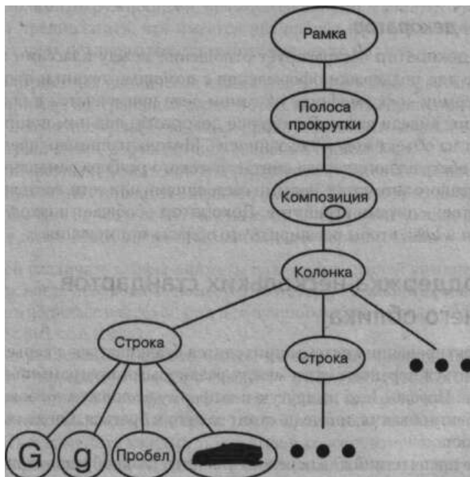
Рис. 2.8. Объектная структура после добавления элементов оформления
