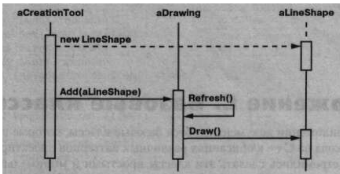
Рис. В.3. Нотация диаграмм взаимодействия
